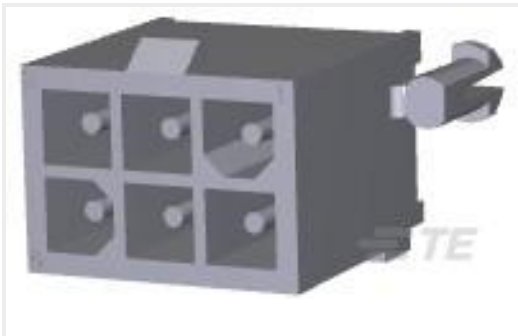
TE Part #1-770875-1 06P MINI UMNL HDR ASSY AU LF
